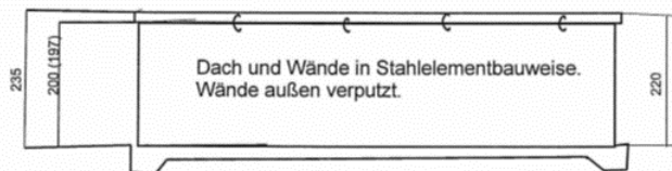
Querschnitt
