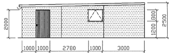
Seitenansicht links
